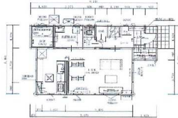
1階 平面図 3.11/200
